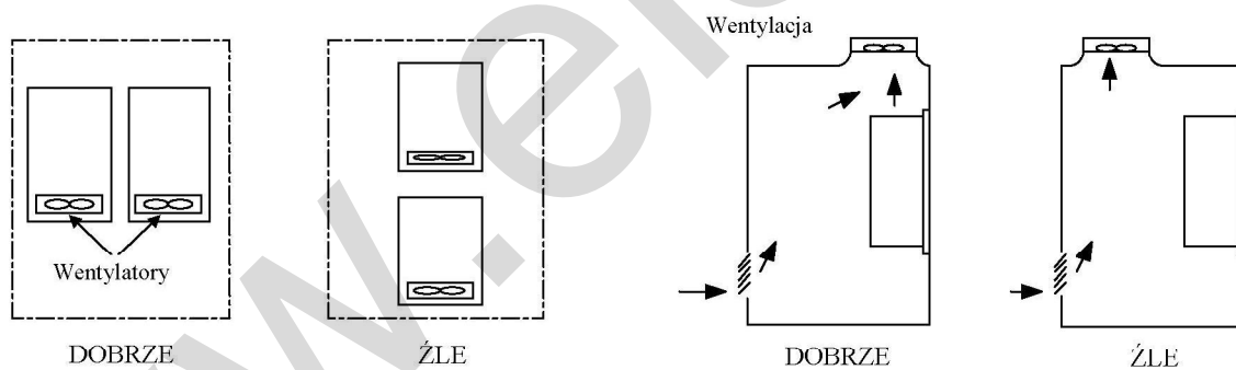
Umieszczenie kilku falowników w szafie
