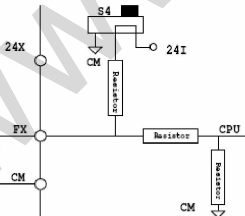
(NPN) Użycie napięcia wewnętrznego falownika
